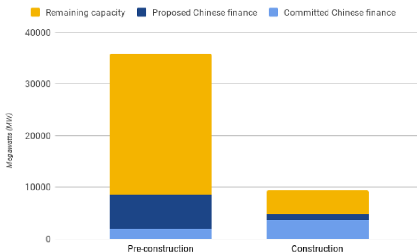
Hình 6. Công suất các nhà máy nhiệt điện than được Trung Quốc tài trợ đang xây dựng ở Việt Nam (MW)
