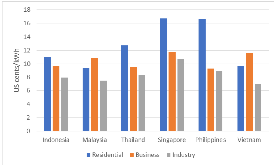
Hình 3: So sánh giá bán điện giữa các quốc gia Đông Nam Á, 2018
