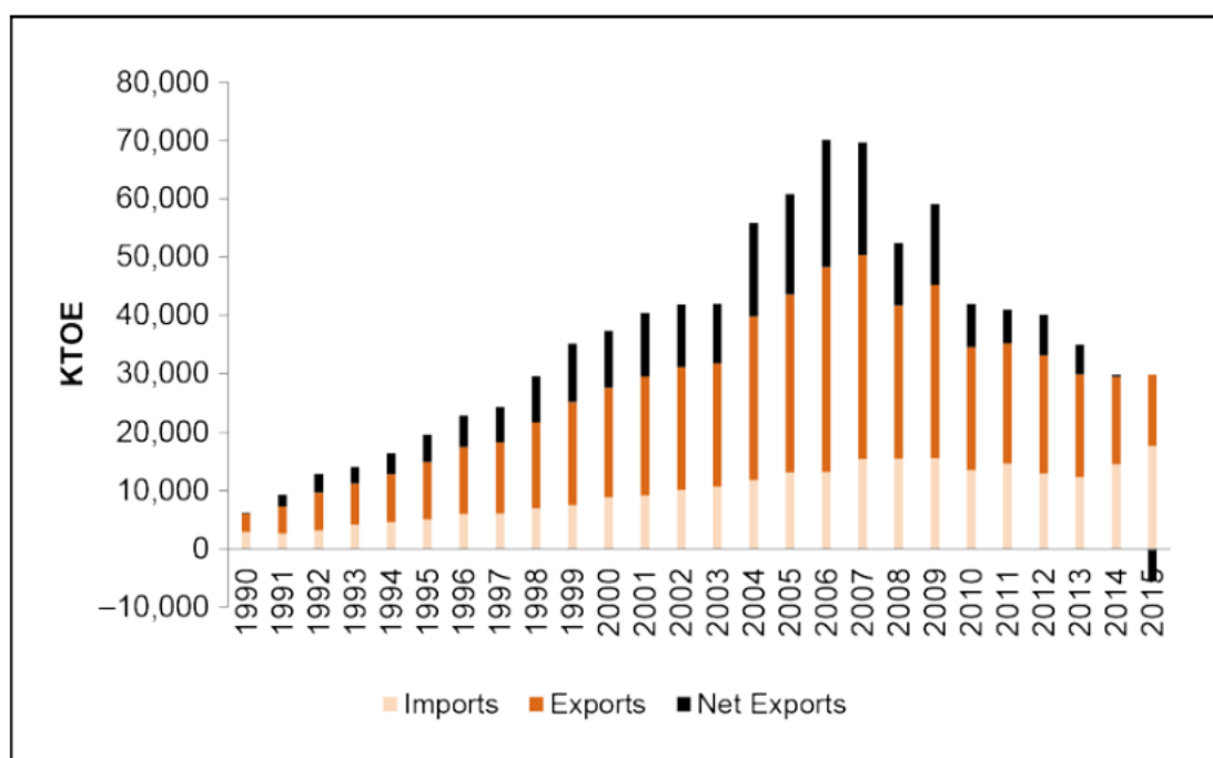
Hình 5: Cán cân xuất - nhập khẩu năng lượng của Việt Nam
