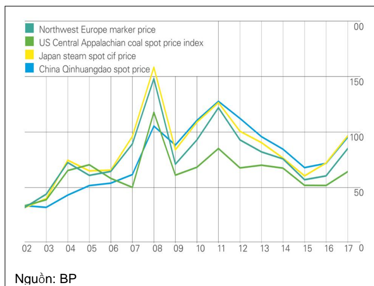
Hình 3: Giá than trên thị trường giao ngay (USD/tấn)
