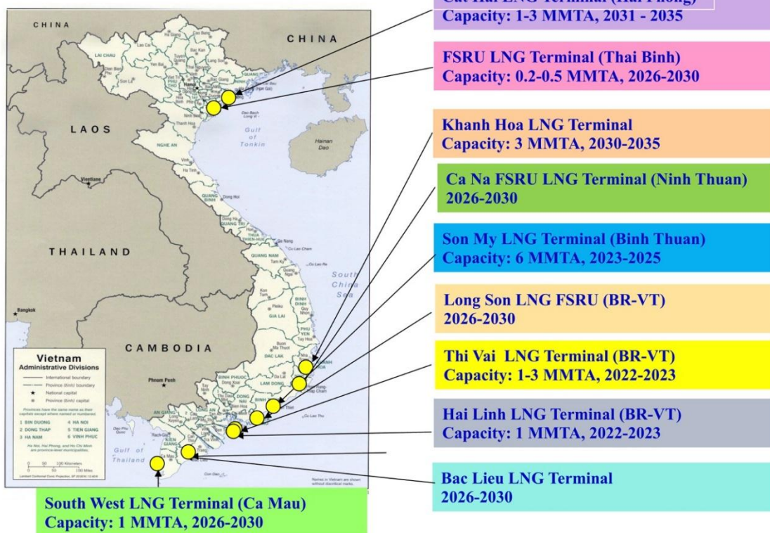
Hình 1. Hệ thống đầu cuối khí thiên nhiên được đề xuất hoặc đang xây dựng, 2019.
